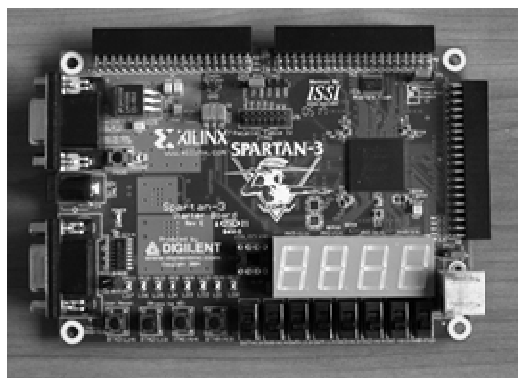
Rys. 3. Płyta z układem FPGA Spartan3.
