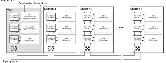
Rys. 1. Schemat blokowy systemu przetwarzania rozproszonego.
