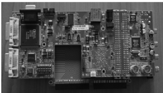
Rys. 2. Zdjęcie płyty VSK (Video Starter Kit) z układem Virtex II.
