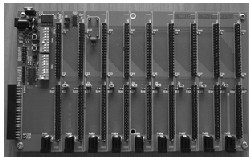
Rys. 4. Płyta bazowa ze slotami łączącymi wszystkie moduły.
